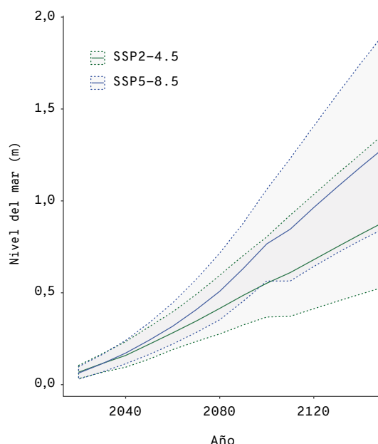
Figura 2. Proyecciones de la subida del nivel del mar Mediterráneo entre los años 2010 y 2150 según el sexto informe del IPCC 6-8 para las trayectorias socioeconómicas compartidas SSP2-4,5 y SSP5-8,5. Las líneas discontinuas muestran los intervalos de confianza de cambio probable (percentiles 17 y 83). FUENTE: Sexto informe del IPCC. 6-8
