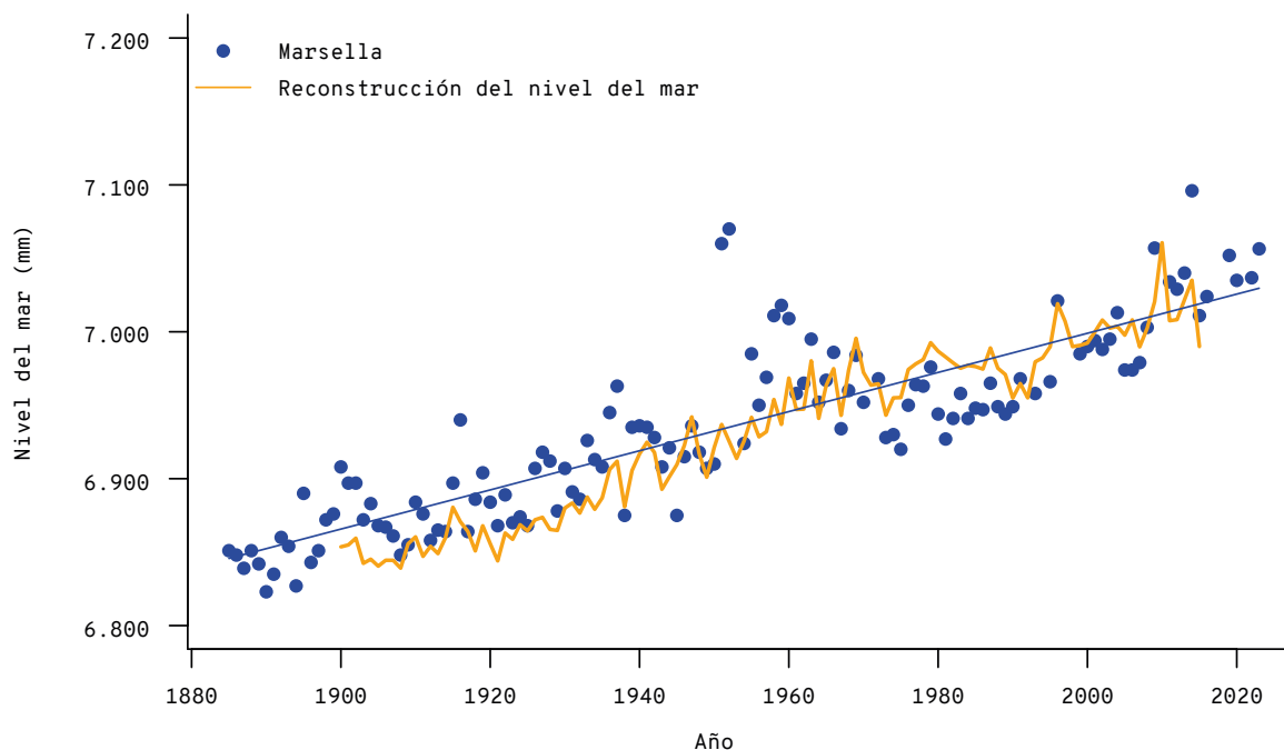
Figura 1. Media anual del nivel del mar en la estación de Marsella. La línea azul muestra el ajuste de una regresión lineal. Para el período entre 1885 y 2023, la estación de Marsella ha mostrado un aumento del nivel del mar de 1,33 \pm 0,07 mm/año ( R^2 = 0,74 ; p < 0,0001 ). La línea de color naranja muestra una reconstrucción de la media del nivel de mar del Mediterráneo occidental entre los años 1900 y 2015 calculada por Dangendorf y colaboradores. 1 FUENTE: PSMSL y Universidad de Hawái. 4-5
